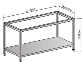
Bordunderstell
